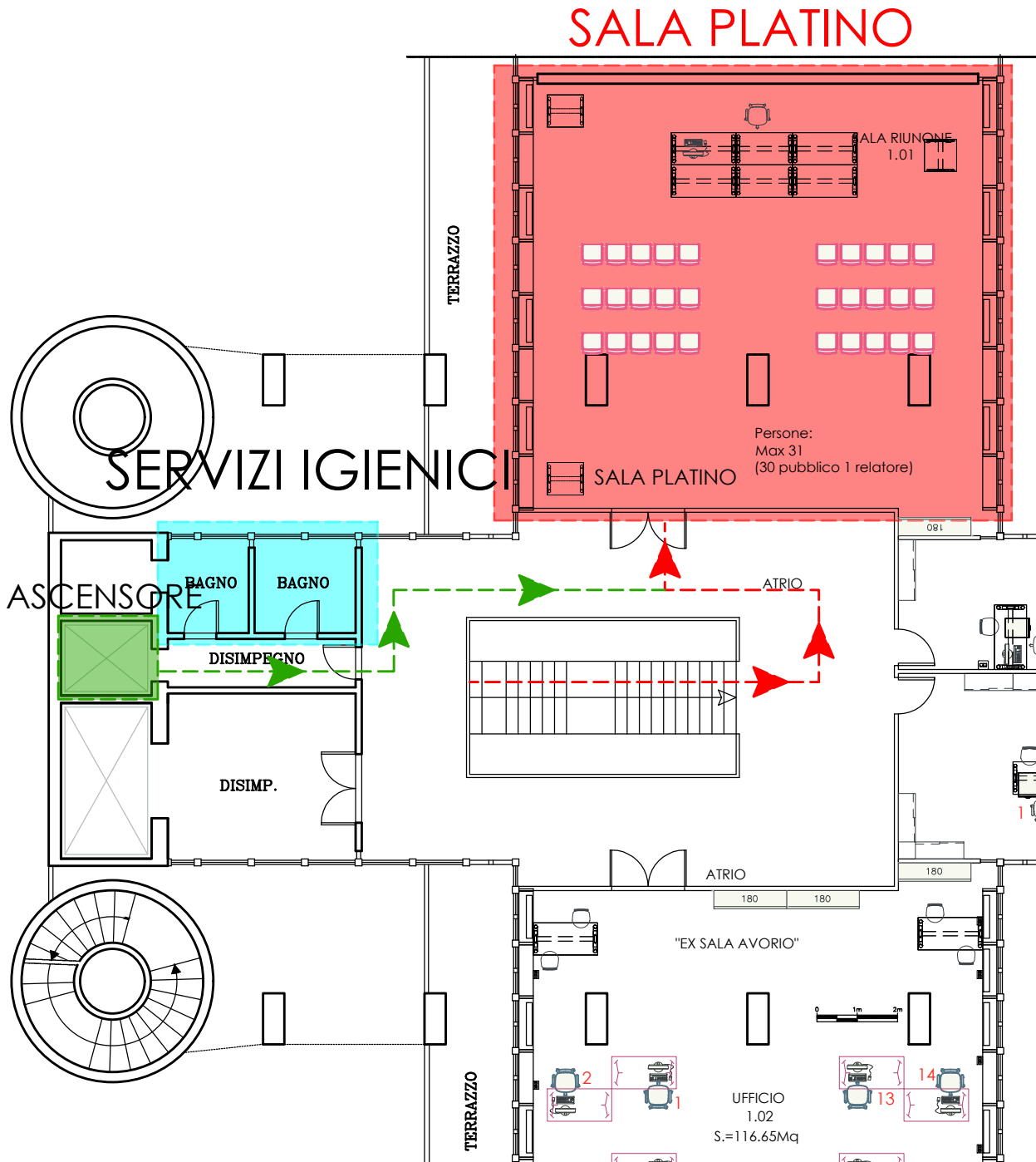
PIANO AMMEZZATO
